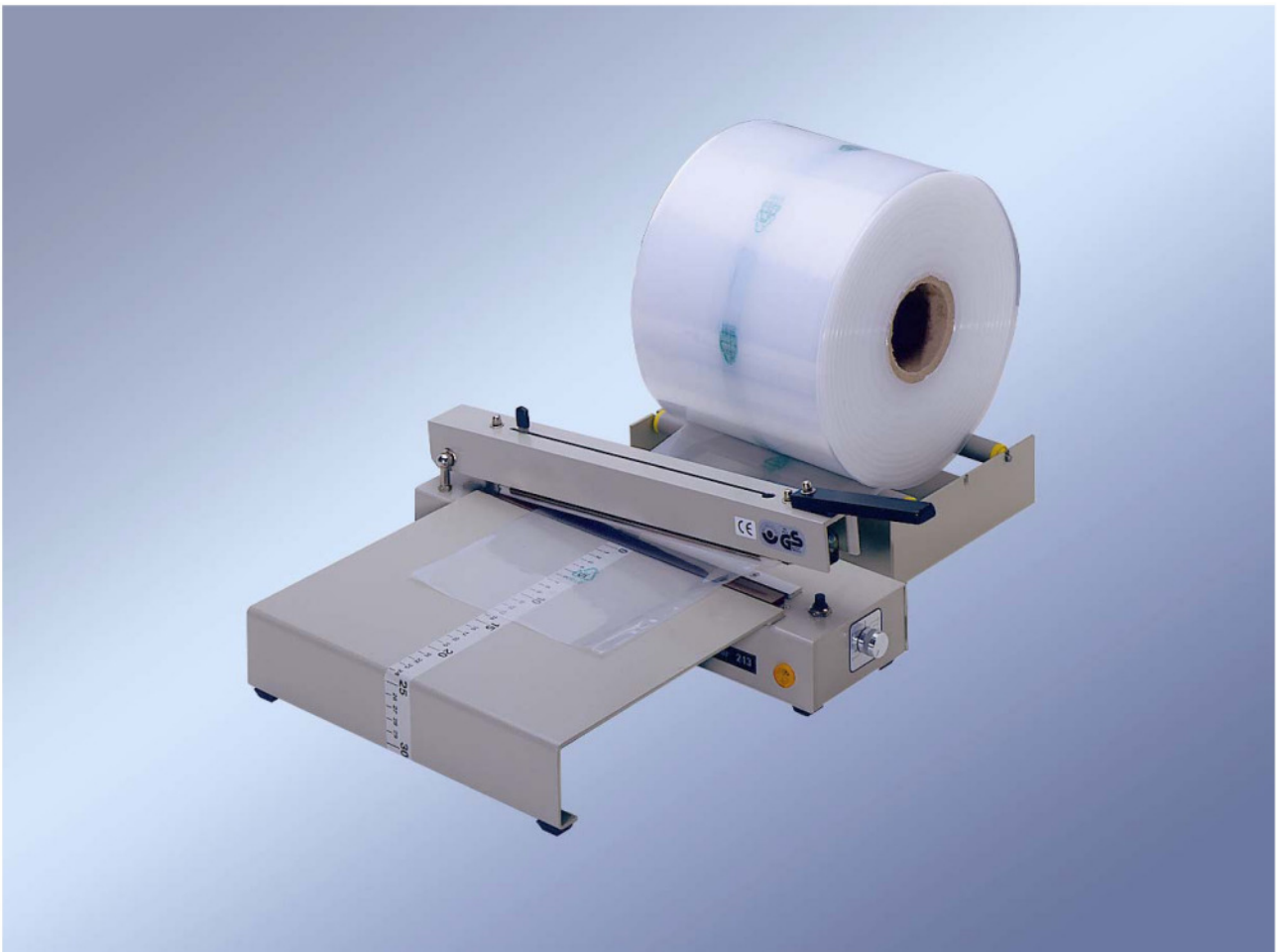
polystar® 243 mit Schneidvorrichtung (SV), Anstecktisch und Folienabroller
